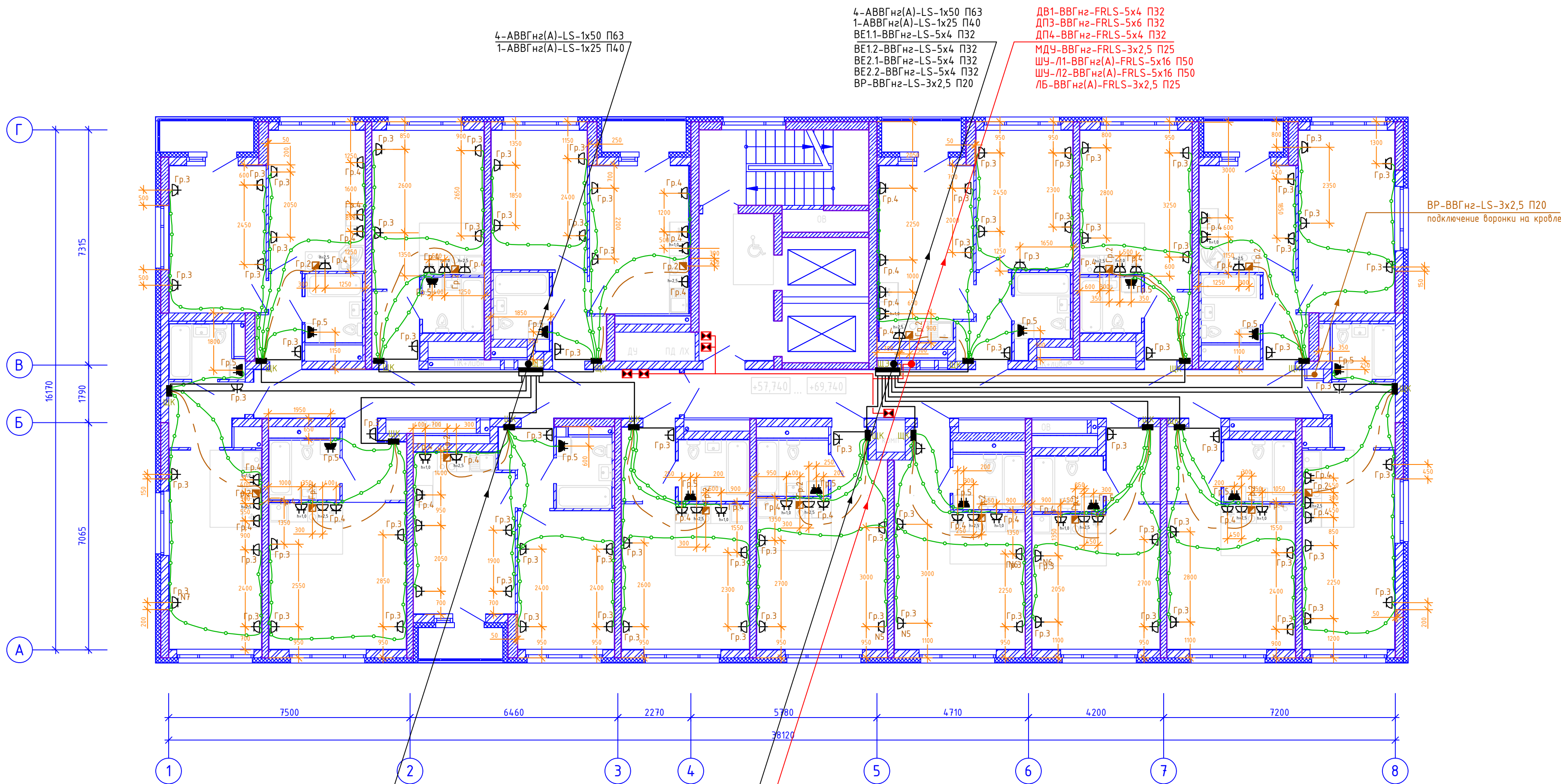
План 20-24этажа
