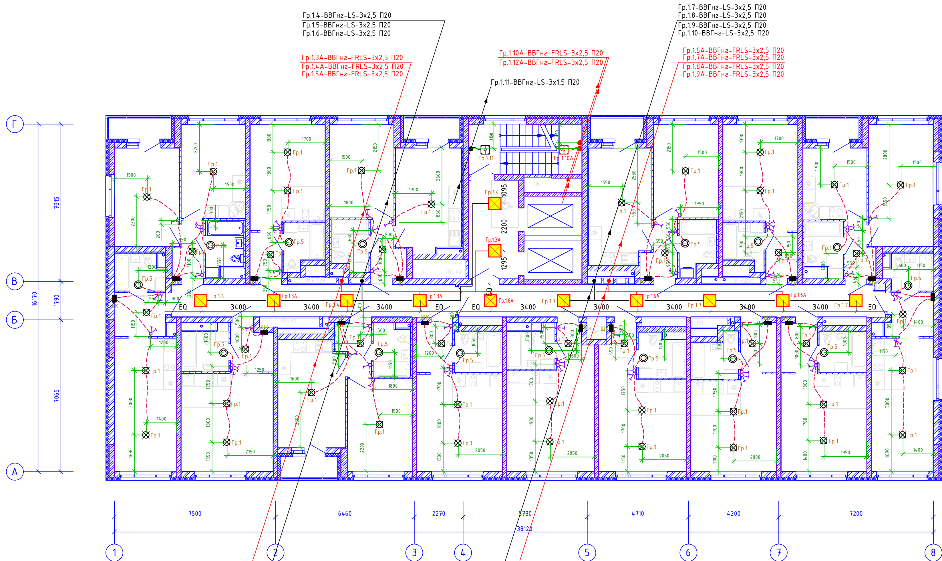
План 3 этажа
